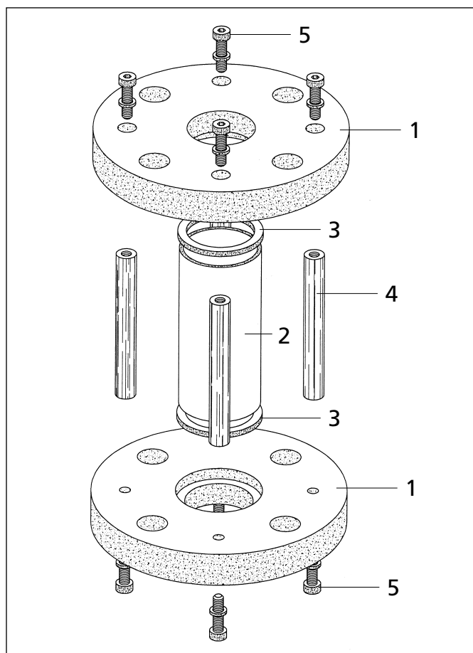
Aufbau einer Lumiglas Durchfluss-Schauglas-Armatur
